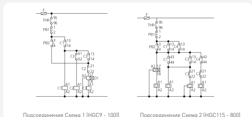
Подсоединение Схема 1 (HGC9 - 100)
