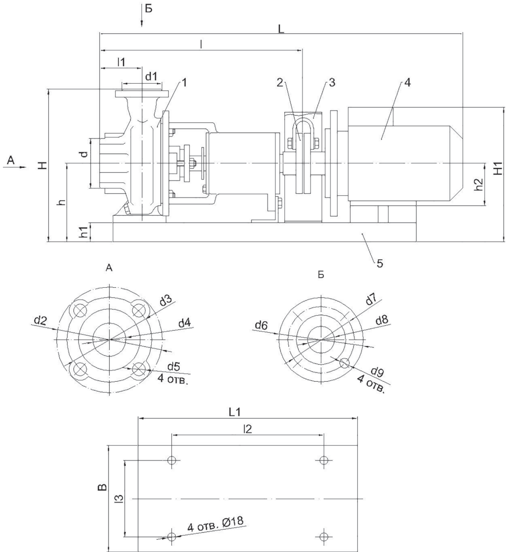
Рис.2 Габаритные и присоединительные размеры насоса 1 - насос; 2 - муфта; 3 - кожух; 4 - электродвигатель; 5 - плата
