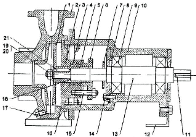
Рис.3 Разрез насоса
